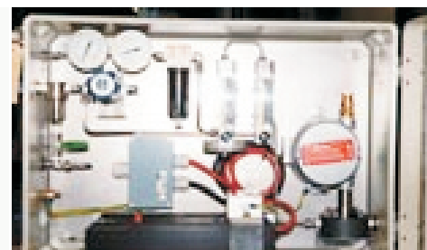
• Sulfurex® - wbudowany pomiar H 2 S oraz system pobierania próbek
